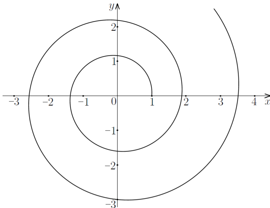
Рис. 12: График функции r = ae^{m\varphi}
